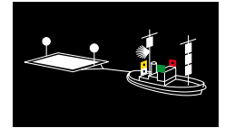
Schleppverbände in Fahrt; Links: bis 200m Schleplänge (Schlepper nicht über 50m Länge); Mitte: mit längsseits geschleppten Anhängen; Rechts: über 200m Länge, mit außergewöhnlichem Schwimmkörper (schleppendes Fahrzeug über 50m lang)
